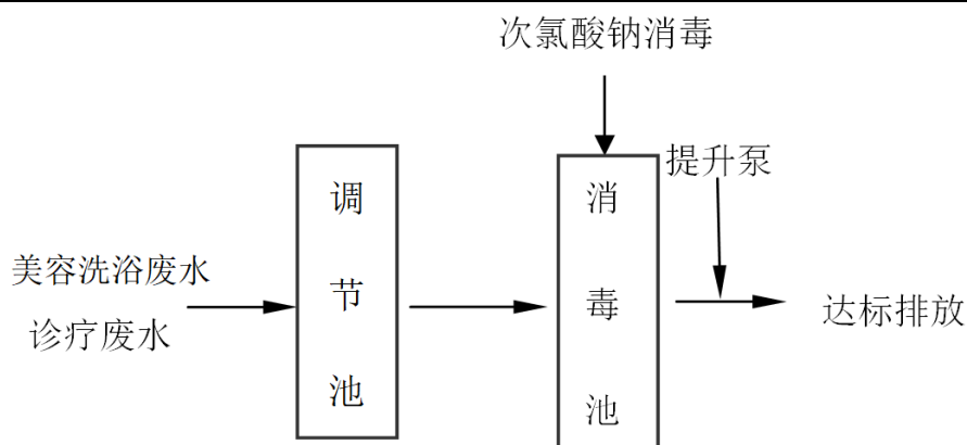
图 6 项目污水处理工艺流程图
