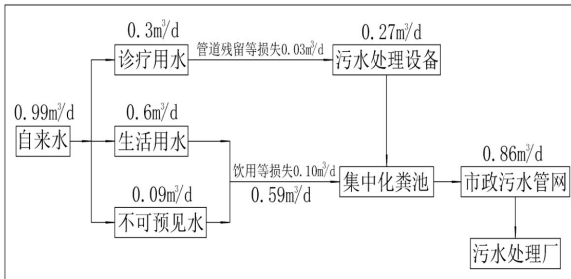
图 3 项目水平衡图
